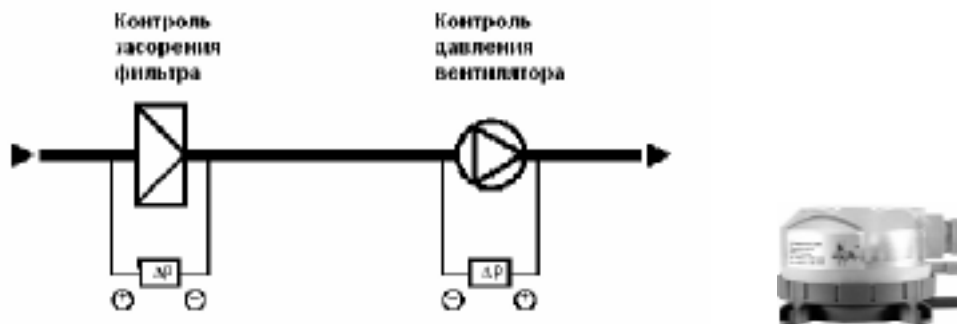
Рисунок 4. Внешний вид и примеры использования датчиков давления.
