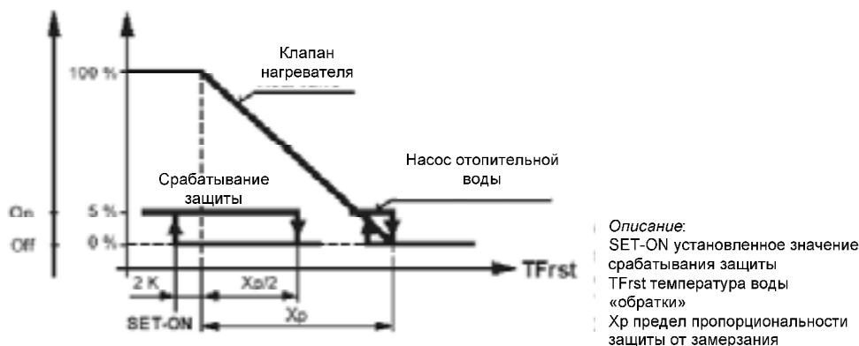
Рисунок 3. Активная защита от замерзания.
