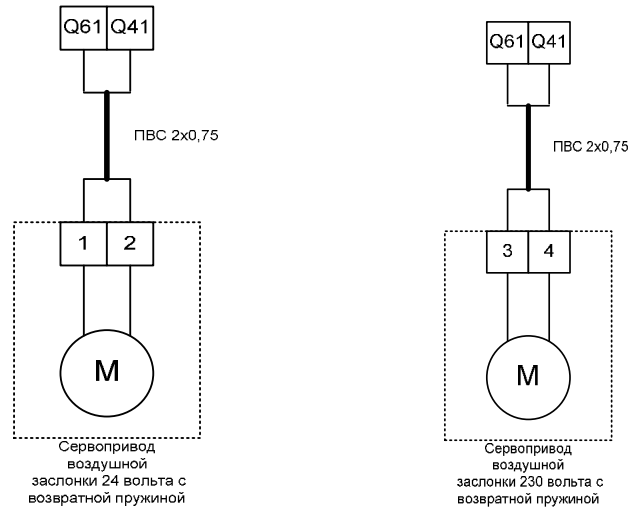
Рисунок 5. Подключение заслонок наружного воздуха.
